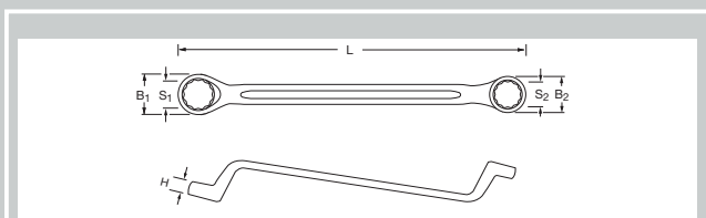
SlimLine očkové klíče, jednotlivé
